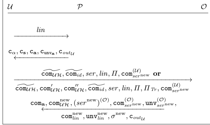
Fig. 37: Message overview for \pi -Update.
