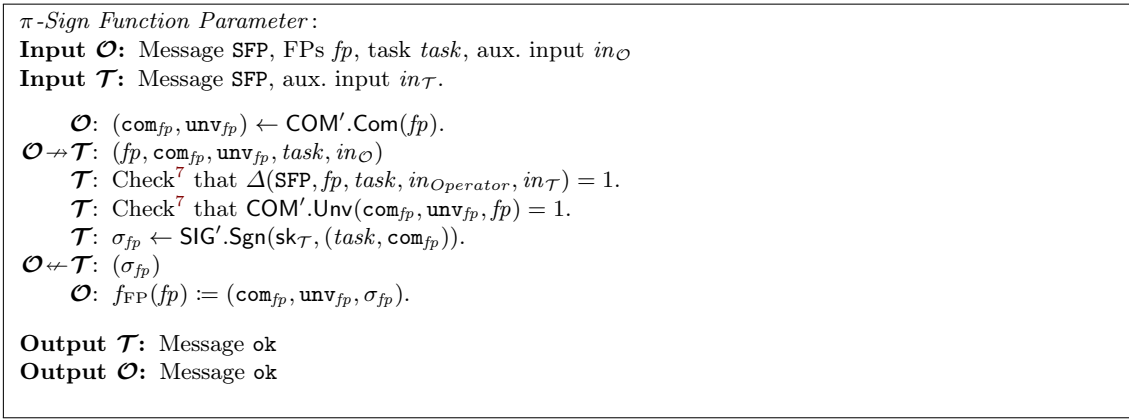
Fig. 22: The protocol \pi -Sign Function Parameter for the Sign Function Parameter-task (Fig. 8).
