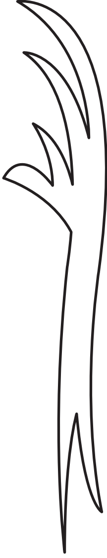
Cirros
