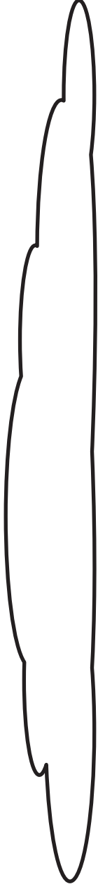
Nimbostratos
