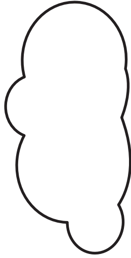
Cúmulos
