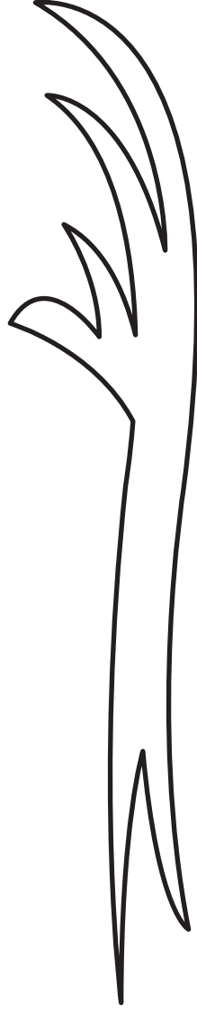
Cirros
