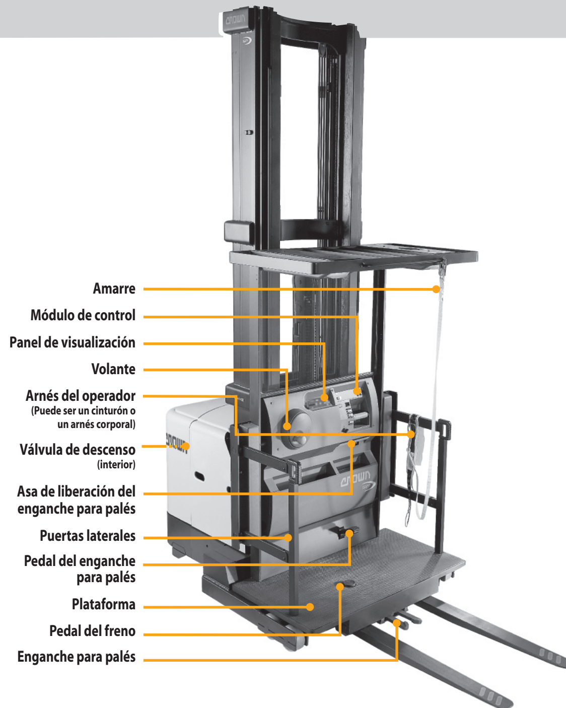
Partes de la carretilla 10
