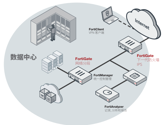
FortiGate 3400E 在数据中心的部署 (IPS / NGFW, 基于意图的网络分段)
