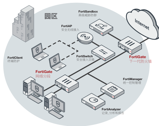
FortiGate 3400E 在园区网络中的部署 (NGFW, 基于意图的网络分段)
