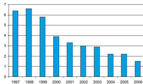
4.11.10.2 Årlige middelkonsentrasjoner av sum PAH i luft på Zeppelifjellet. Enhet: ng/m 3 . Den årlige middelkonsentrasjonen av PAH har hatt en klar nedadgående trend i perioden fra 1999 til 2006.
