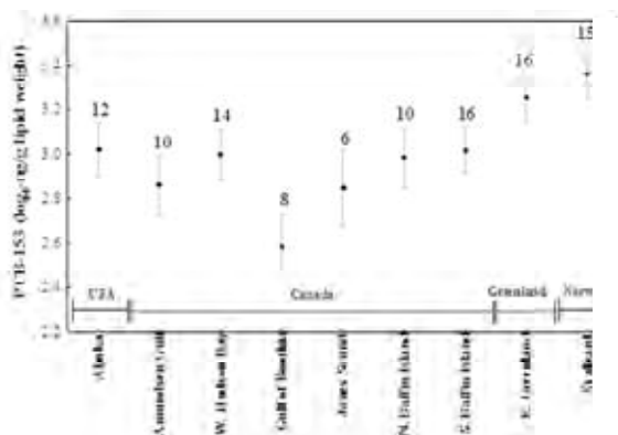
Figur 4.11.1.2 Geografisk fordeling av PCB-153 (ng/g fettvev) i isbjørn fra ni forskjellige populasjoner listet etter lengdegrad fra vest til øst. Middeler verdier er vist med 95 % konfidensintervall. (Fra Verreault et al 2005a).
