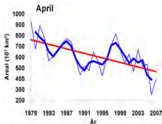
Figur 4.1.1.2. Trender i isutbredelse for april måned. Tynn kurve viser årlige middelveier, tykk viser løpende 3- årsmiddel, og rett linje viser trenden for perioden 1979- 2007.
