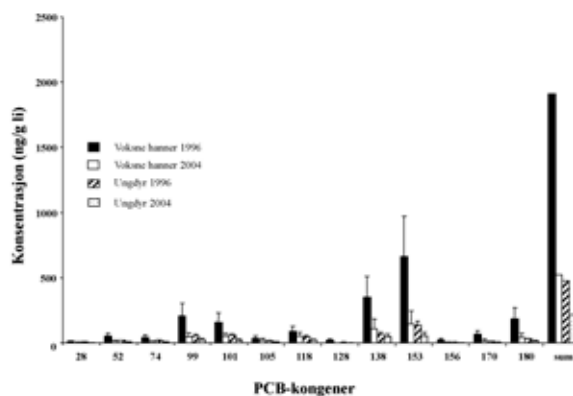
Figur 4.11.2.2 Konsentrasjon av PCB-konsentrasjoner (alle kongener) (ng/g ekstraherbart lipid) i spekk fra voksne hanner og ungdyr av ringsel. Kongsfjorden, Svalbard 1996 og 2004.
