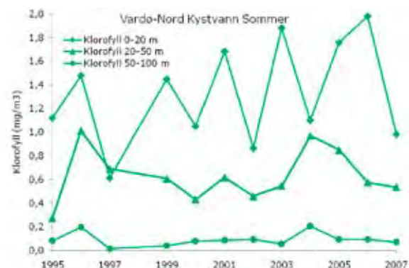
Figur 4.3.1.2. Klorofyll a i tre dybdelag i kystvannet i snittene Fugløya-Bjørnøya (venstre) og Vardø-Nord (høyre) om sommeren (august).
