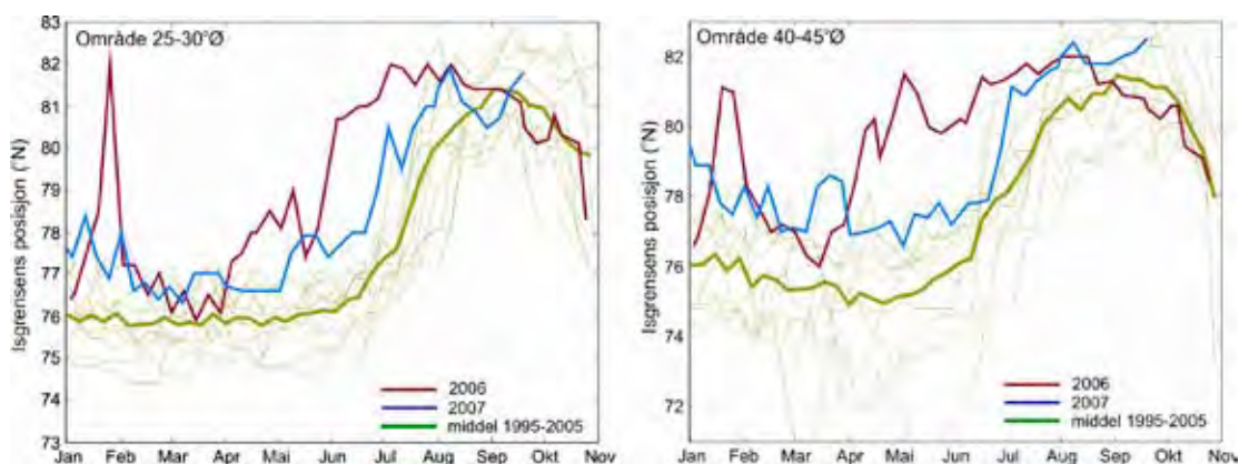
Figur 4.1.1.4. Nordlig posisjon på iskanten i det vestlige (området 25-30oØ) og sentrale (området 40-45oØ) Barentshavet gjennom året. De tynne grønne linjene viser enkeltårene 1995-2005 og den tykke grønne linjen er middelet av disse. Den røde linjen viser isgrensen i 2006 og den blå i 2007.
