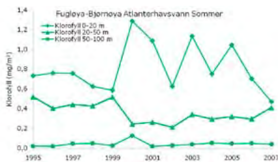
Figur 4.3.1.1. Klorofyll a i tre dybdelag i atlantehavsvannet i snittene Fugløya-Bjørnøya (venstre) og Vardø-Nord (høyre) om sommeren (august).
