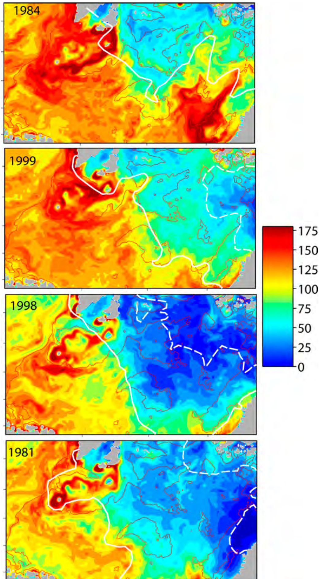
Figur 4.3.1.3. Årlig primærproduksjon i Barentshavet for fire utvalgte år ( \text{g C m}^{-2} \text{år}^{-1} ). Isgrenser angitt for april og september.
