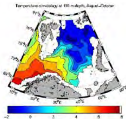
Figur 3.1.1.2 Gjennomsnittlig sommertemperatur i Barentshavet ved 100m dyp. Observasjoner i august – oktober i perioden 1977 – 1979. Polarfronten er skarper hvert enkelt år, men blir spredd i gjennomsnitt.
