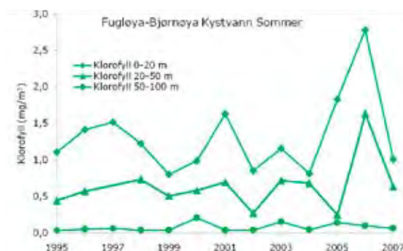
Figur 4.3.1.2. Klorofyll a i tre dybdelag i kystvannet i snittene Fugløya-Bjørnøya (venstre) og Vardø-Nord (høyre) om sommeren (august).
