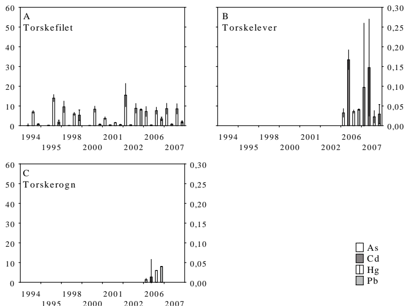
Fig. 4.11.4.5 Konsentrasjoner (gjennomsnitt ± største og minste verdi) fra 1994 til i dag av tungmetallene arsen, kadmi-um, kvikksølv og bly i A) torskemuskel, B) torsk lever og C) torskerogn fra Barentshavet. Torskerogn er analysert i samleprøver, og lever og rogn ble ikke analysert før i 2006.
