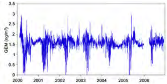
4.11.10.3 Tidsserier for elementært kvikksølv i gass-fase (GEM) ved Zeppelifjellet, 2000-2006. Om våren hvert år opptrer det episoder hvor konsentrasjonen av elementært kvikksølv i gassfase blir sterkt redusert (samtidig med at konsentrasjonen av ozon i luft også blir kraftig redusert). Årsaken er at lys ved polar soloppgang starter en kjemisk prosess som omdanner kvikksølv til mer reaktive komponenter som dermed blir biologisk tilgjengelige.
