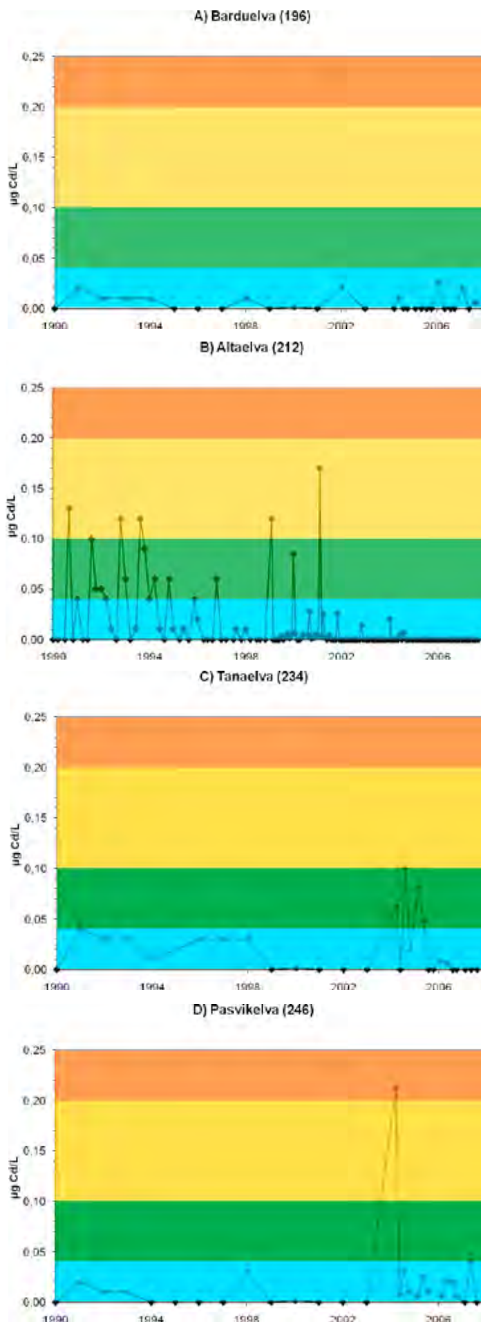
Figur 4.11.11.2 Variasjon i konsentrasjoner av kadmium (Cd, µg/l) i perioden 1990-2007, på RID-stasjonene i Barduelva (A), Altaelva (B), Tana (C) og Pasvikelva (D). Fargekodene angir tilstandsklasser i forhold til SFTs klassifiseringssystem for miljøkvalitet i ferskvann.
