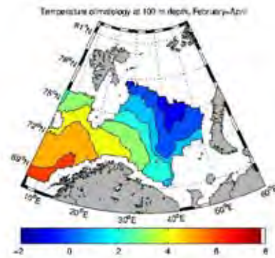
Figur 3.1.1.1 Gjennomsnittlig vintertemperatur i Barentshavet ved 100m dyp. Observasjoner i februar – april i perioden 1977 – 1979. Polarfronten er skarper hvert enkelt år, men blir spredd i gjennomsnitt.
