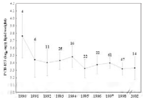
Figur 4.11.1.3 Trend fra 1990 til 2002 av PCB-153 (ng/g fettvev) i isbjørn fra Svalbard målt i plasma. Middeler verdier er vist med 95 % konfidensintervall. (Fra Henriksen et al. 2001).
