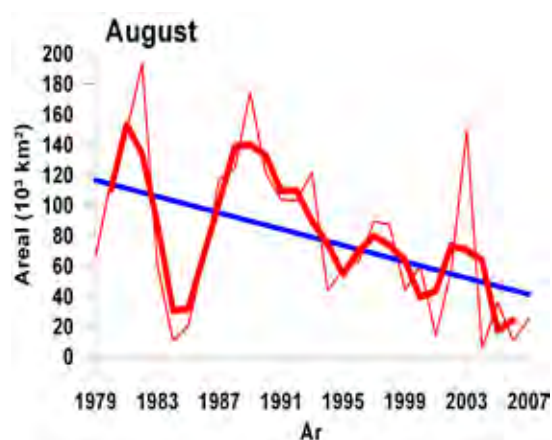
Figur 4.1.1.3. Trender i isutbredelse for august måned. Tynn kurve viser årlige middelveier, tykk viser løpende 3- årsmiddel, og rett linje viser trenden for perioden 1979- 2007.
