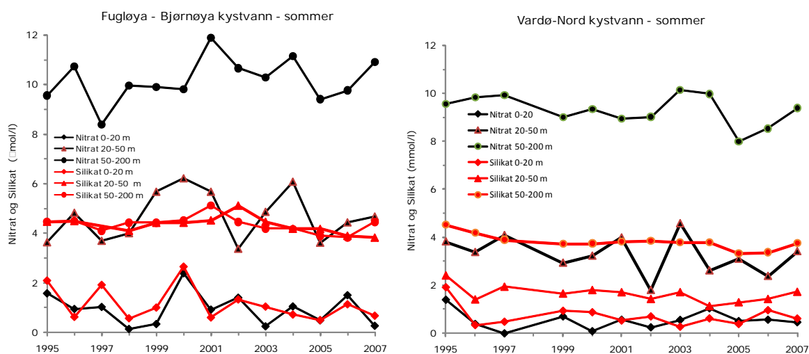
Figur 4.1.2.5. Næringsalter i tre dybdelag i Kystvannet i snittene Fugløya-Bjørnøya (venstre) og Vardø-Nord (høyre) om sommeren (august).
