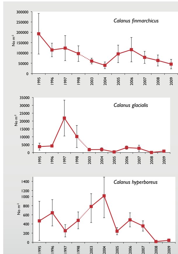
Figur 4.4.2.1 Årlig gjennomsnittlig forekomst av hoppekrepsene Calanus finmarchicus , C. glacialis , og C. hyperboreus på Fugløya–Bjørnøya-snittet (4 stasjoner) i perioden 1995–1998 og 2003–2009.
