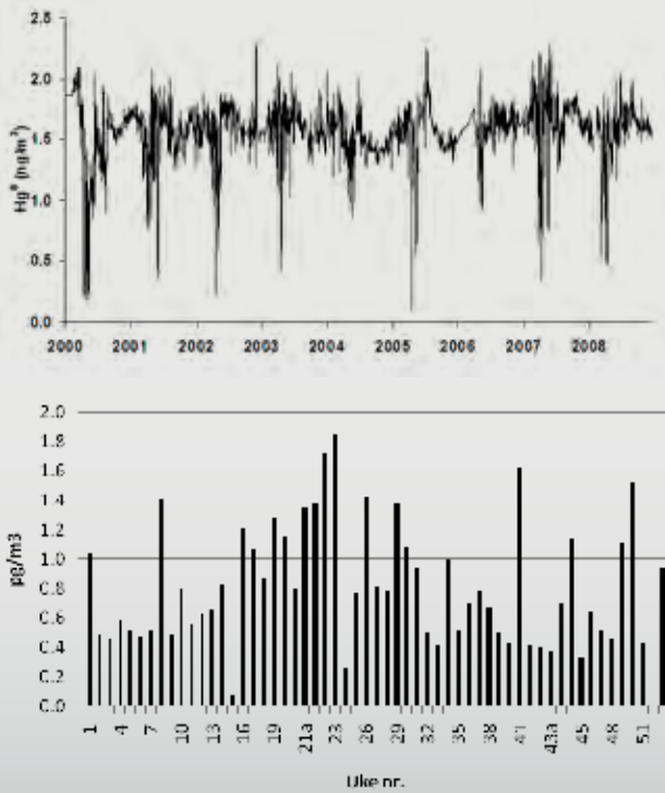
Figur 4.11.2.4 Tidsserier for elementært kvikksølv i gassfase (GEM) ved Zeppelinfjell, 2000-2008. Hver vår opptrer det episoder hvor konsentrasjonen av elementært kvikksølv i gassfase blir sterkt redusert samtidig med at konsentrasjonen av ozon i luft også blir kraftig redusert. Årsaken er at lys ved polar soloppgang starter en kjemisk prosess som omdanner kvikksølv til mer reaktive komponenter som dermed blir biotilgjengelige.
