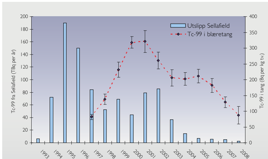
Figur 4.11.8.2 Tidsserie for ^{99}\text{Tc} i blæretang fra Hillesøy ( \text{Bq kg}^{-1} tørrvekt) i perioden 1997-2008.
