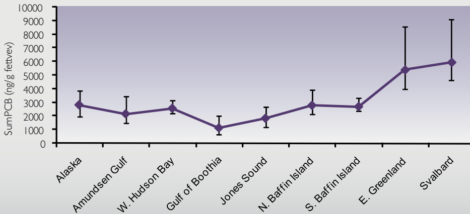
Figur 4.11.6.5 Geografisk fordeling av PCB (sum av 42 PCB-forbindelser) (ng/g fettvev) i isbjørn (hunnar) fra ni forskjellige populasjoner listet etter lengdegrad fra vest til øst. Middelerdier er vist med \pm 95 % konfidensintervall (Fra Verreault et al. 2005).
