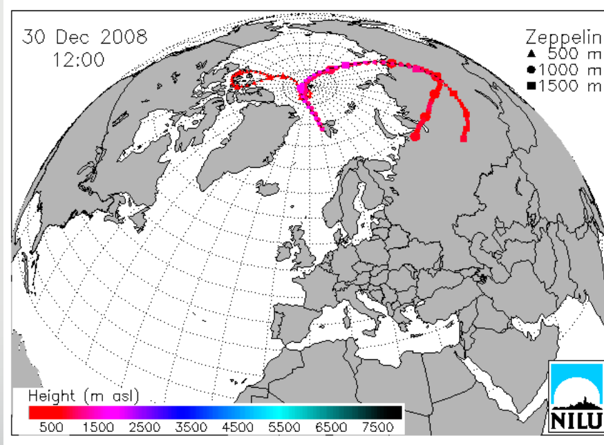
Figur 4.11.2.3 Beregnete trajektorier med adkomst til Zeppelin-observatoriet under prøvetaking av prøven med høyest verdi for sum PAH i 2008. Figuren viser tydelig transportveien for de mest forurensete luftmassene.
