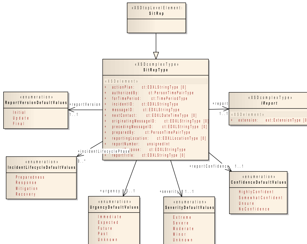
Figure 3: EDXLSitRepRoot Elements
