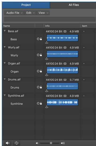
Project Browser
