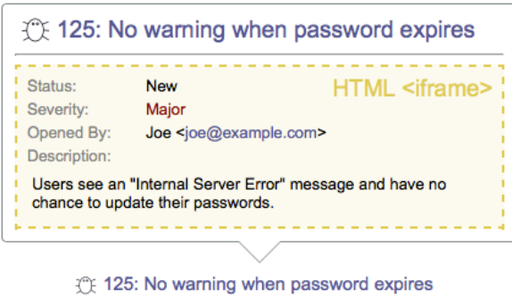
Fig. 2 Preview iframe
