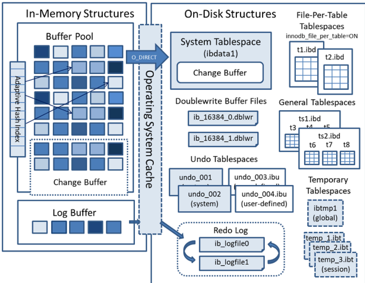
図 15.1 InnoDB のアーキテクチャ
