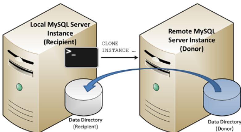
図 5.2 リモートクローニング操作
