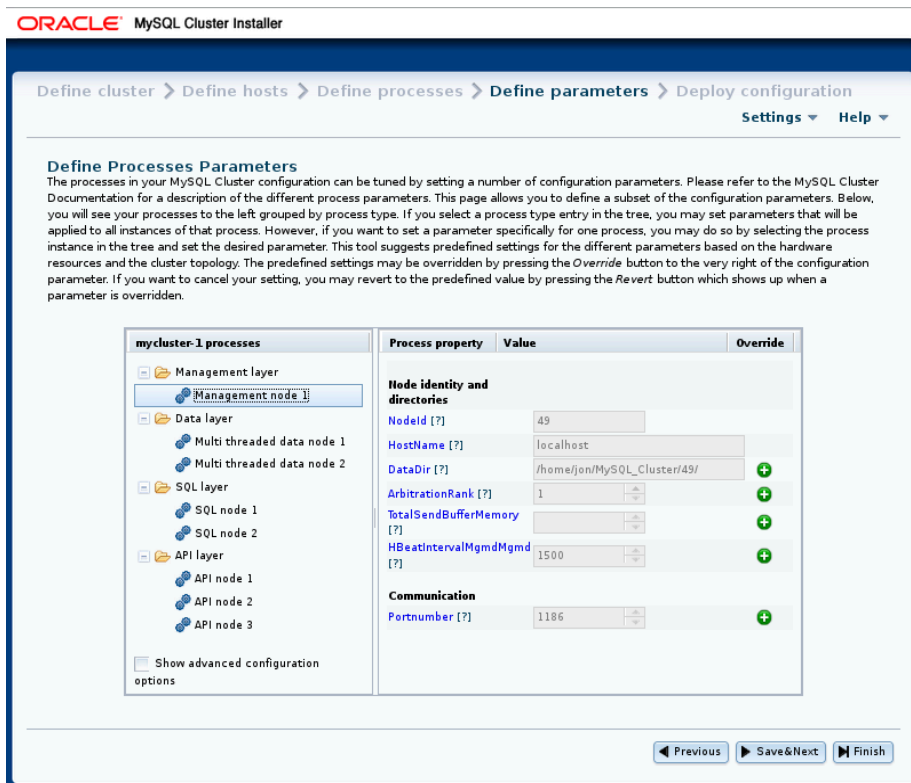
図 23.19 パラメータの定義 - プロセス属性
