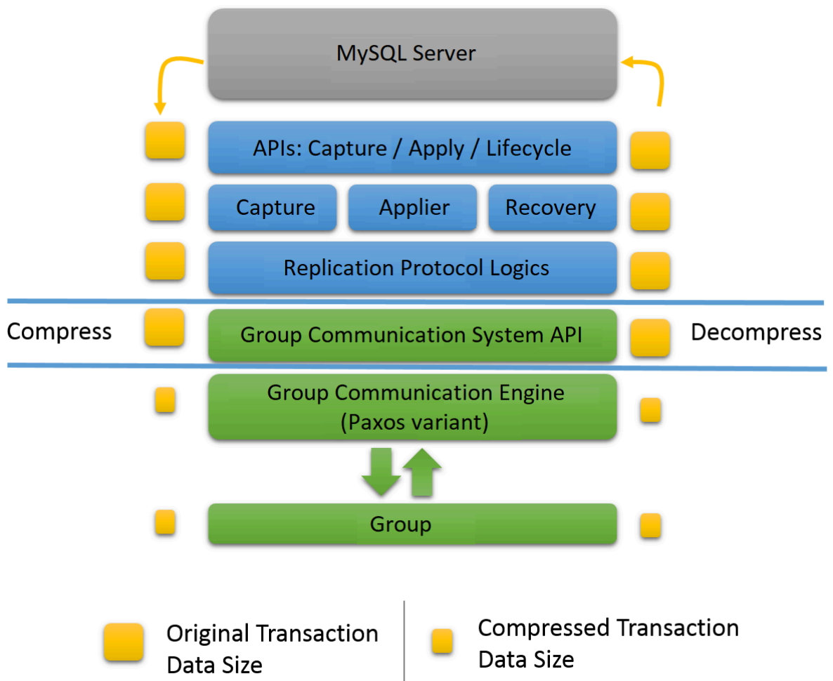
図 18.15 圧縮のサポート
