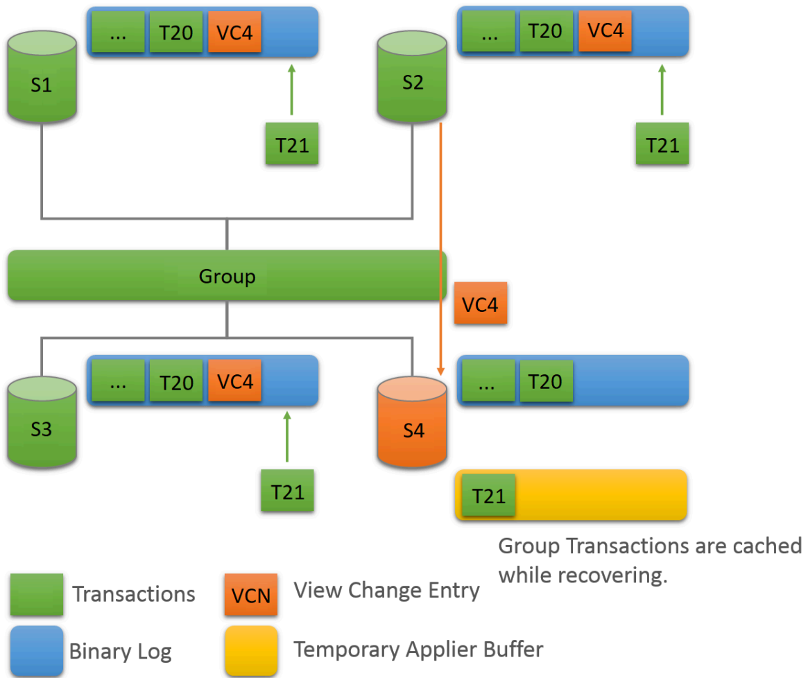
図 18.11 キュー済トランザクション
