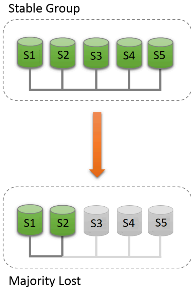
図 18.13 損失クォーラム
