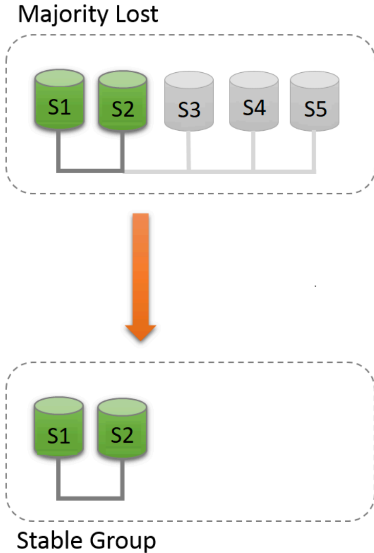
図 18.14 新規メンバーシップの強制
