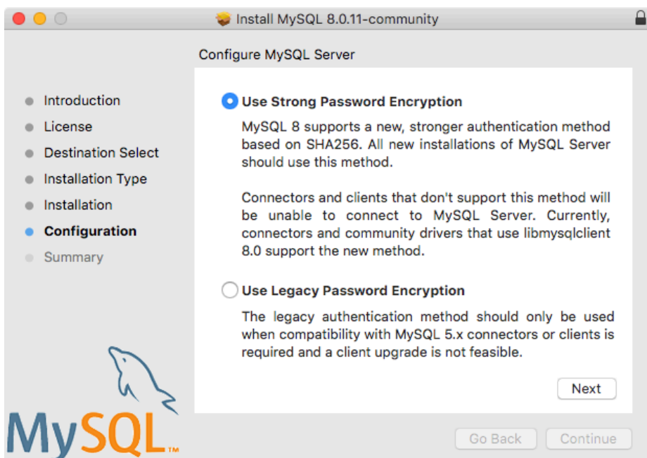
図 2.15 MySQL パッケージインストーラウィザード: パスワード暗号化タイプの選択
