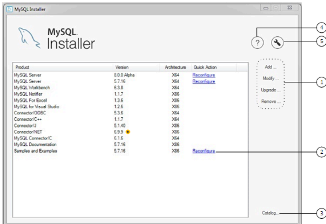
図 2.11 MySQL Installer ダッシュボードの要素
