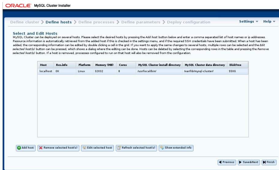
図 23.12 「NDB Cluster ホストの定義」画面, start
