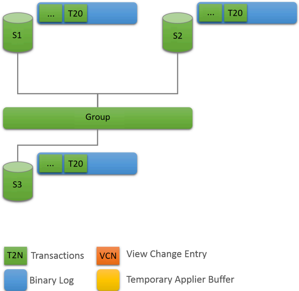
図 18.8 安定グループ
