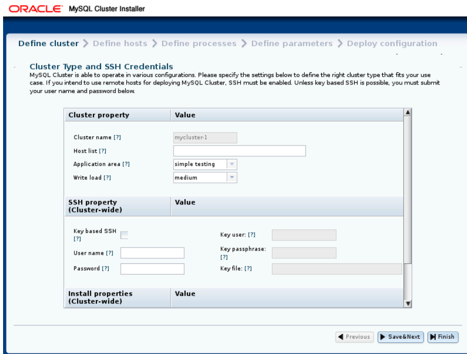
図 23.10 「NDB Cluster 自動インストーラクラスタの定義」画面
