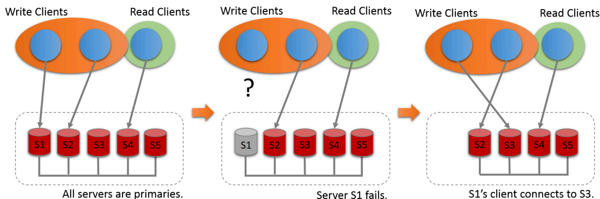
図 18.5 クライアントフェイルオーバー
