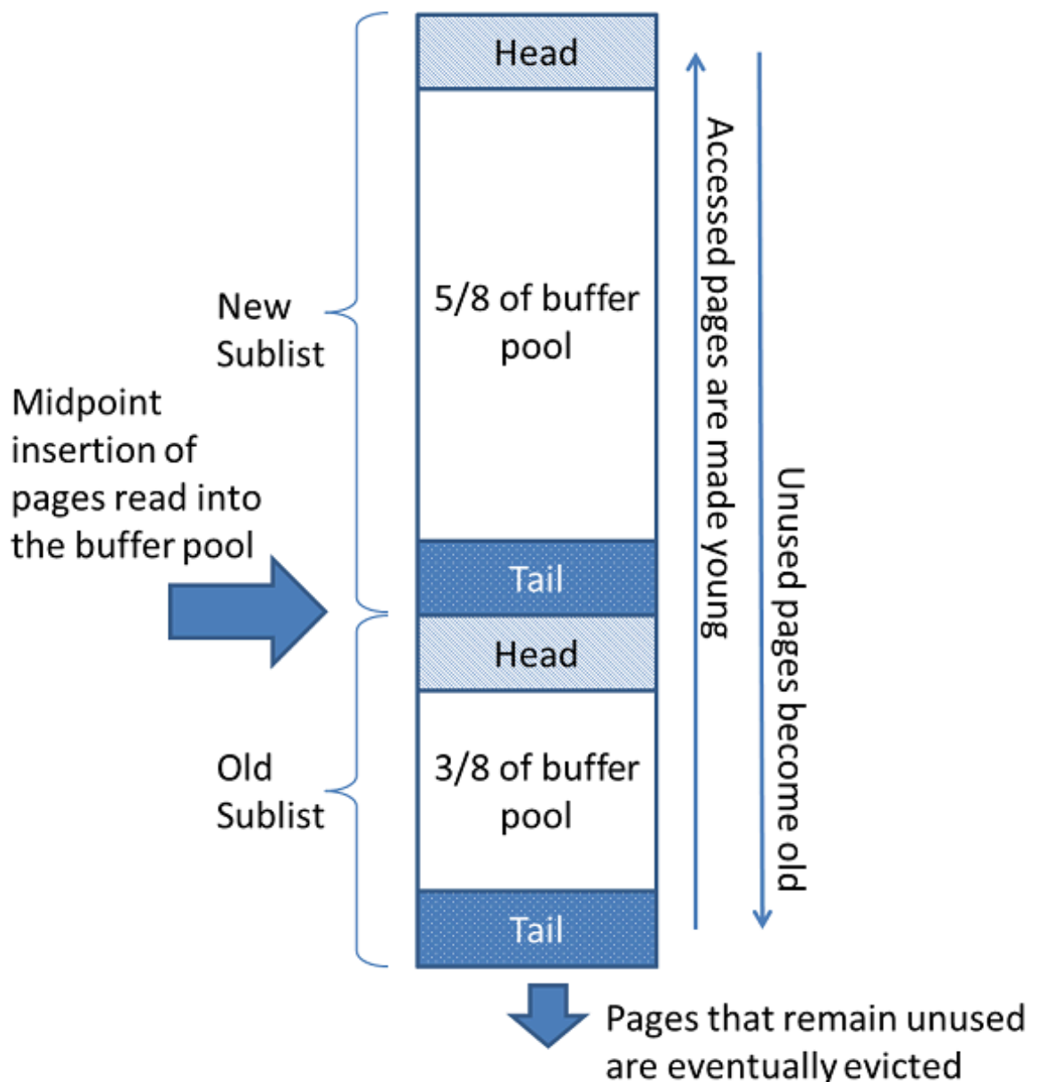
図 15.2 バッファプールリスト
