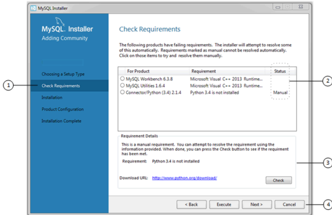
図 2.8 要件のチェック
