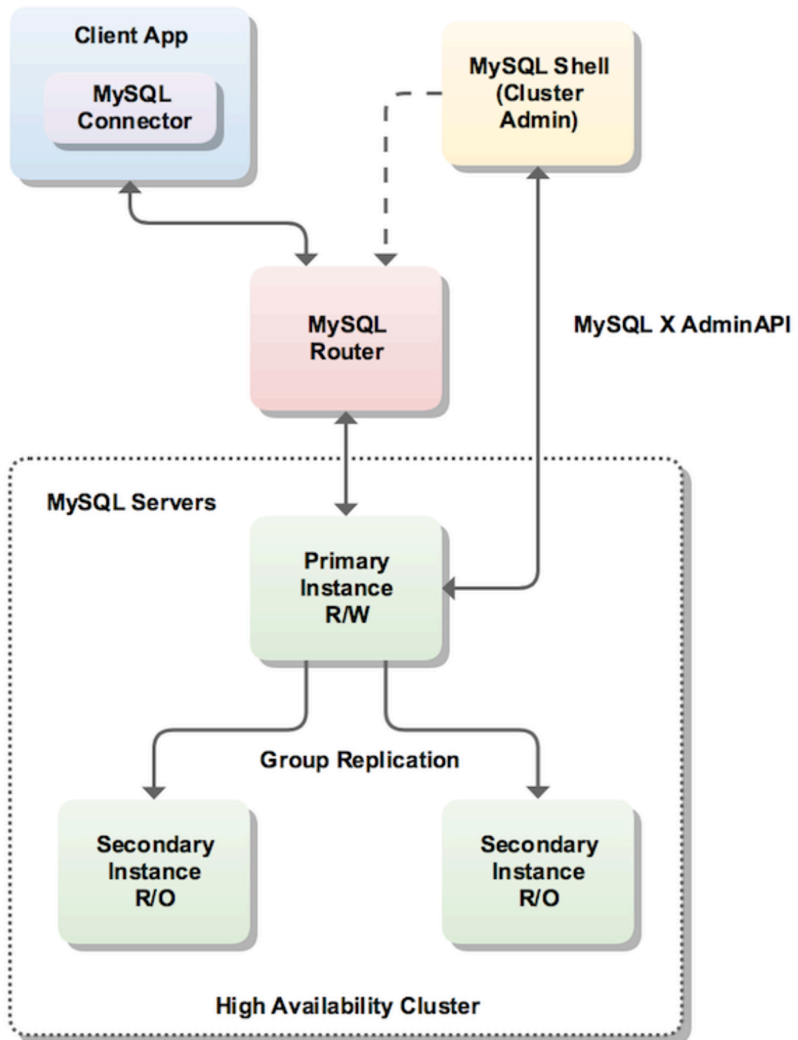
図 21.1 InnoDB クラスターの概要
