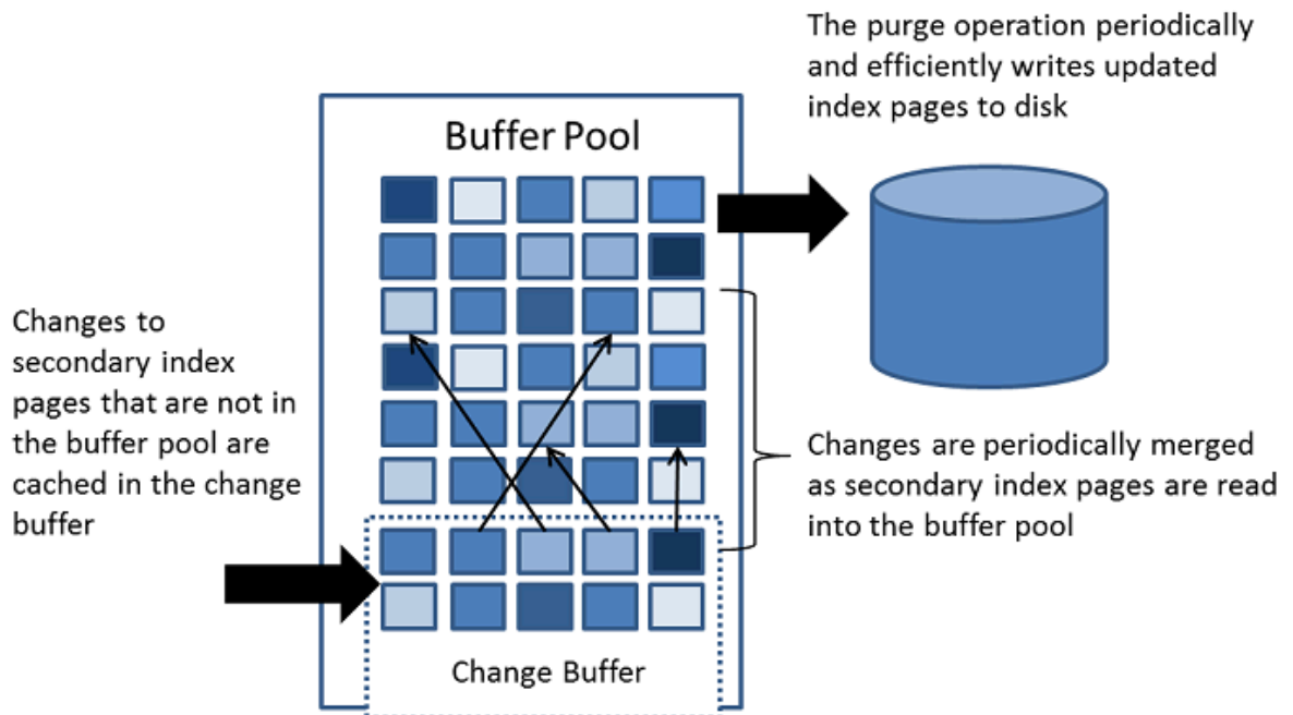
図 15.3 変更バッファ
