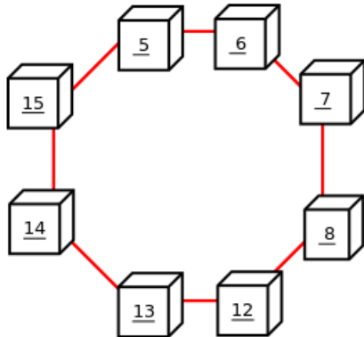
図 23.27 NDB Cluster ノードの循環配置
