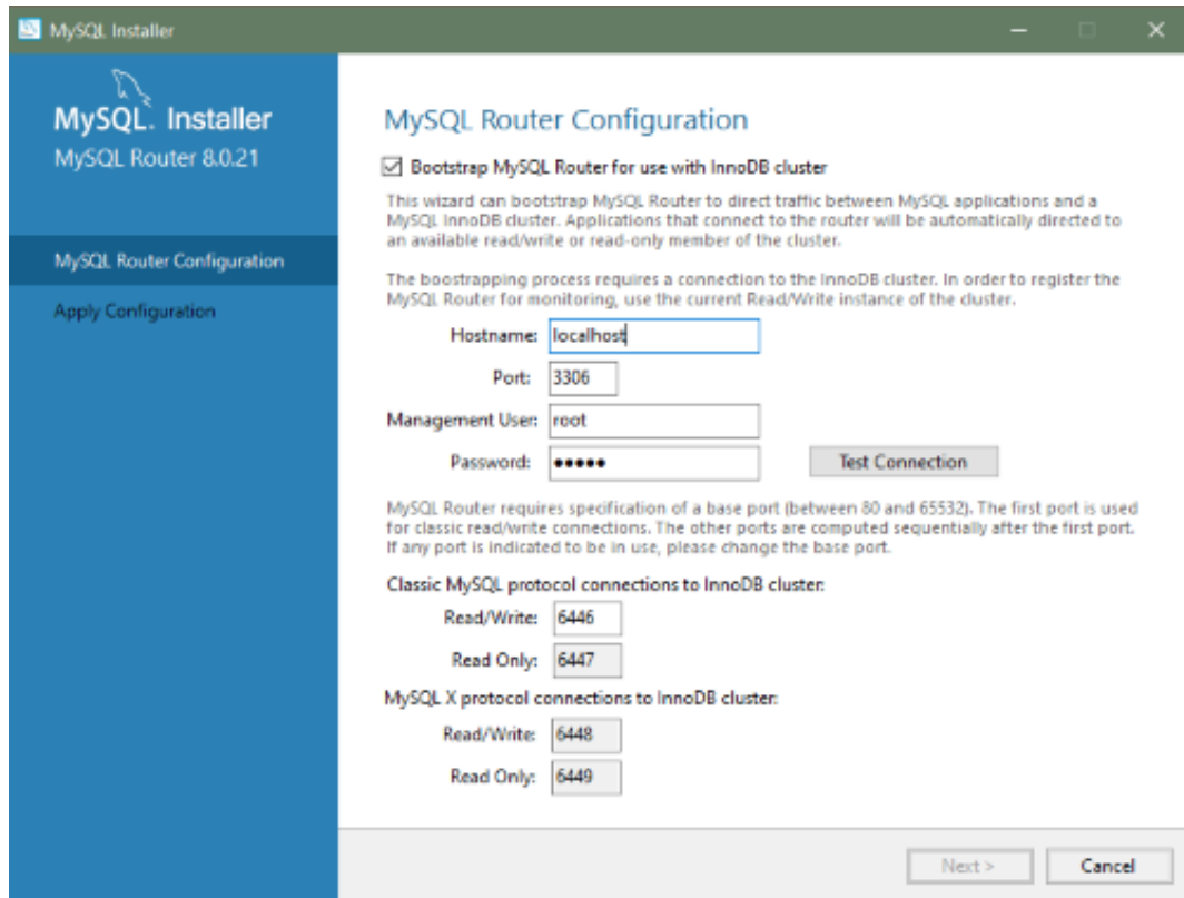
図 2.10 MySQL Router 構成
