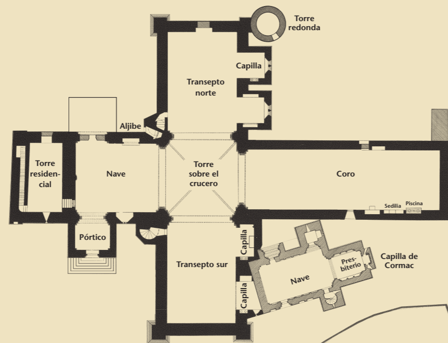
Plano de la planta de la Catedral
