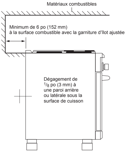
Dégagements pour l'installation en présence d'un dossieret (vendu séparément)
