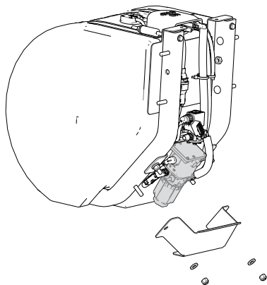
Figura 10: Tanque DEF mediano y grande
