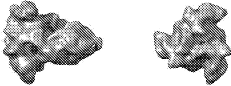
FIG. 14D OC43 S-2P
