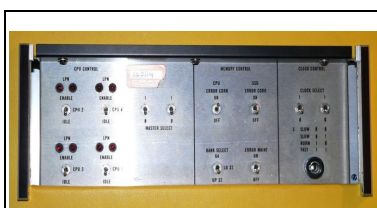
Pannello di controllo del CRAY-XMP48
