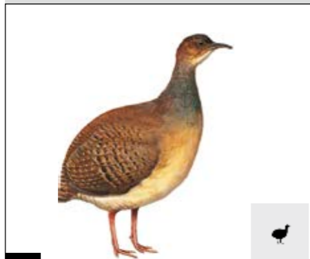
27 Crypturellus erythropus * ♀ ♂
