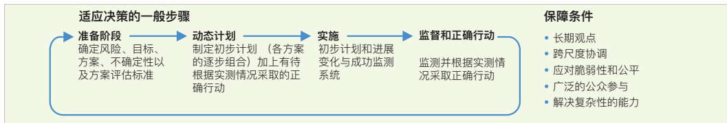
图SPM.5 | c, d
