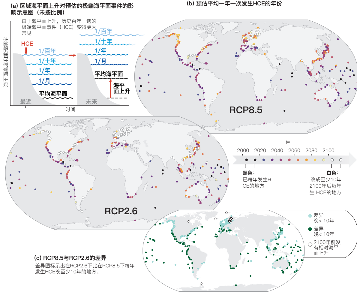
图SPM.4 | 区域海平面上升对沿海各地点极端海平面事件的影响。 (a) 近期（1986–2005）和未来极端海平面事件及其平均重现情况示意图。由于平均海平面上升，历史上每百年发生一次（历史上百年一遇事件，HCE）的局部海平面在未来将更频繁地发生。(b) 观测记录充足的439个沿海地点在RCP8.5和RCP2.6下预计平均每年发生一次HCE的年份。没有圆圈表示由于缺少数据而无法进行评估，但并不表示没有暴露度和风险。圆圈颜色越深，预期这种转变越早。对于预计在2100年之前出现这种转变的地点，可能区间为±10年。白色圆圈（在RCP2.6下有33%的地点，在RCP8.5下有10%的地点）表示预计在2100年之前不会每年发生HCE。(c) 关于在RCP2.6下预估哪些地点HCE转为年度事件的时间比在RCP8.5下晚10年以上的分布图。鉴于各情景会导致到2050年在许多地点出现微小的差异，因此，图中未标示在RCP4.5下的结果，但可参见第4章所述。[4.2.3, 图4.10, 图4.12]
