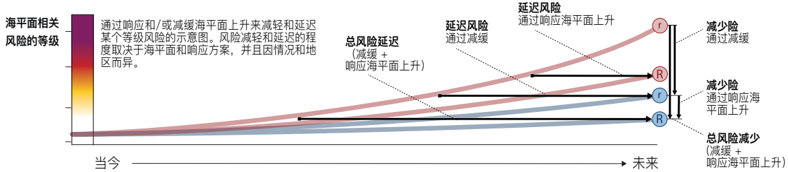
图SPM.5 | a, b
