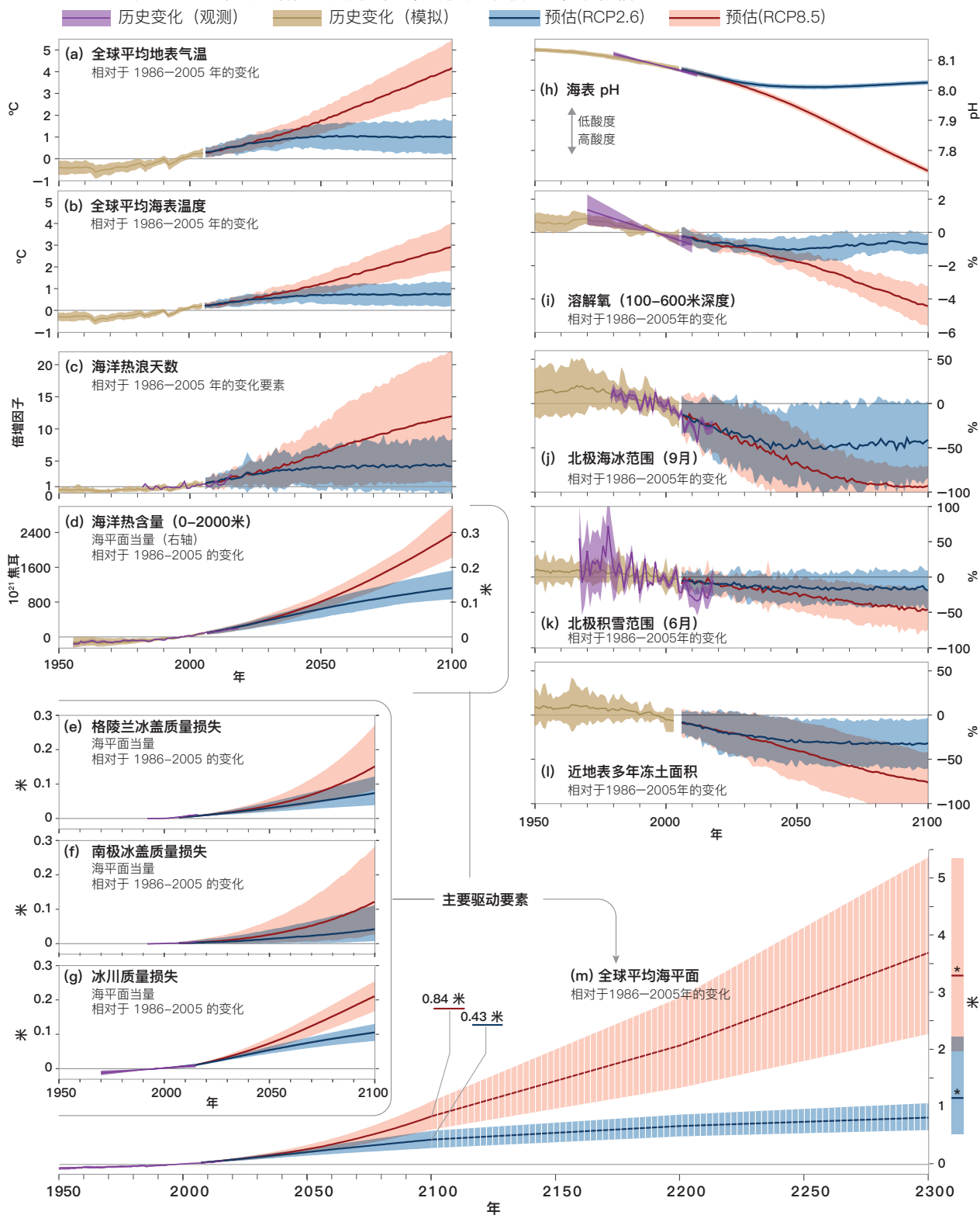
图SPM.1 | 观测到的和模拟的自1950年 11 以来海洋和冰冻圈的历史变化，以及在低（RCP2.6）和高（RCP8.5）温室气体排放情景下预估的未来变化。
