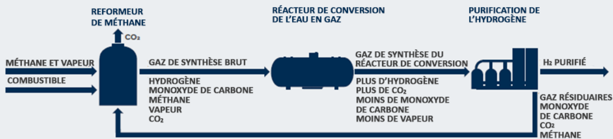
Figure 14 – Procédé de reformage du méthane à la vapeur et description 2
