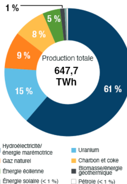
Figure 28 – Production d'électricité par type de carburant au Canada, 2018 (source : Régie de l'énergie du Canada)
